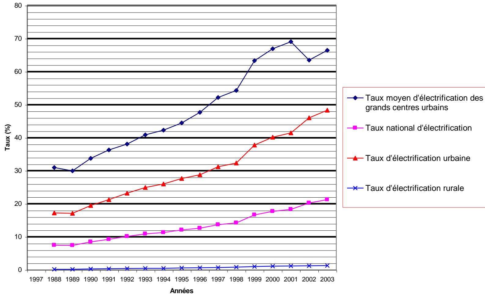
Figure 7 : Evolution du taux d'électrification
